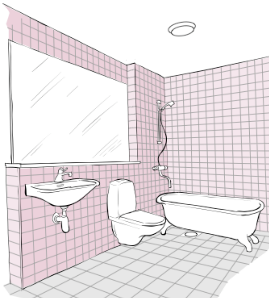
Bild 3b: Våtrumsvägg med installationer som sätts framför betongvägg. Rörinstallationer ska inte fästas styvt i betongväggen. Formination, använd bilden från våtrums-ROT-broschyren
