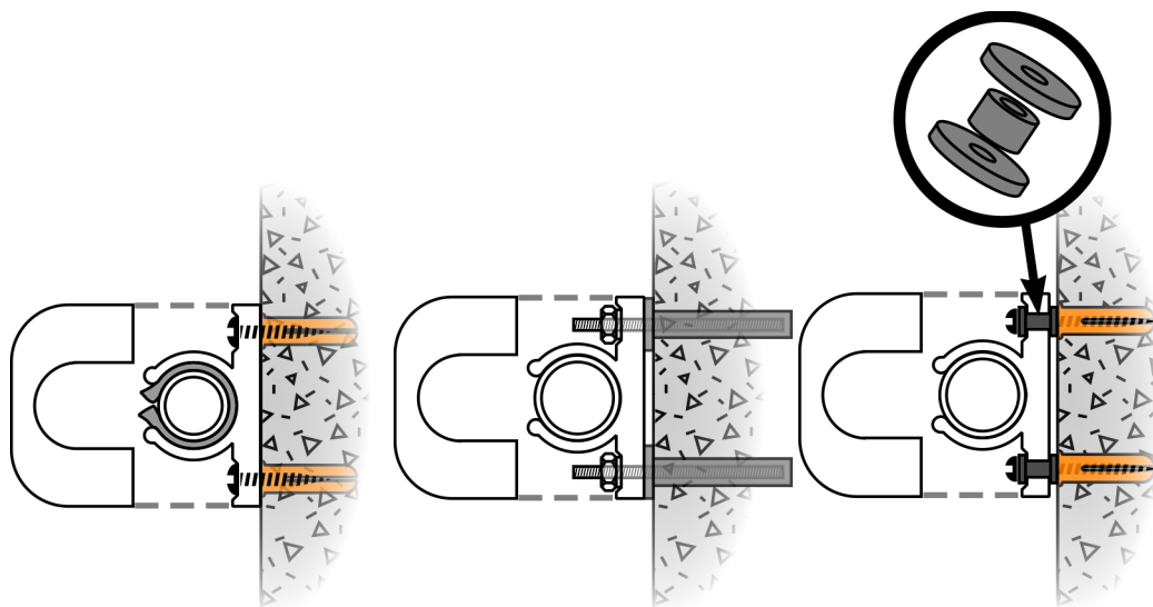
Bild 11. Tre sätt att dämpa stomljud från vatten- och värmerör: a) ljudtejp 2 mm runt röret sätts in i en större klammer (eller innanför ett svep), b) klammer sätts med elastiska stomljudspluggar i betongväggen. c) gummipackning mellan klammer och vägg. Följ rekommendationerna från Säker Vatteninstallation för tätning av infästningar i väggar med tätskikt.
