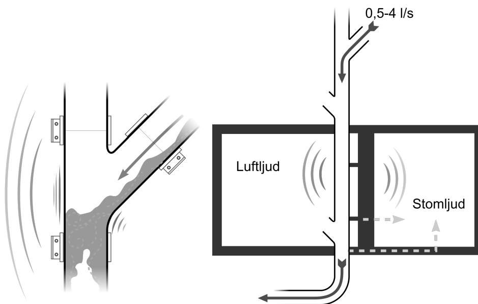
Bild 2. a) I avloppsrör är det strömmande vatten som slår emot förgreningar och dimensionsändringar som ger vibrationer i rörväggarna, b) vibrationerna skapar både
