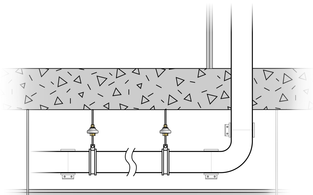
Bild 3a. Bygg in rör i schakt eller ovanför ljudisolerande undertak. Använd vibrationsisolerande och stomljudsisolerande produkter vid upphängning av rör i bjälklag eller vägg då de vetter mot en bostad eller lokal med ljudkrav.
