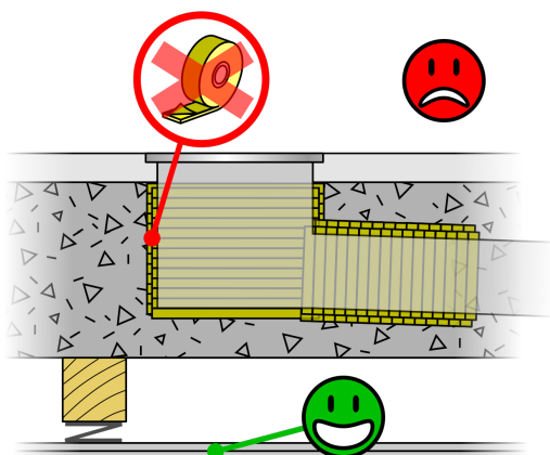
Bild 6. Vid montering av brunn och avloppsrör i bjälklag ovanför sovrum, vardagsrum, matrum och övriga rum med ljudkrav: a) Brunnen bör inte avvibreras utvändigt därför att rörelserna kan medföra läckage i tätskiktet. Välj istället en brunnprodukt som ger lågt stomljud (exempelvis i belagt gjutjärn med plastinsats) eller tilläggsisolera undersidan av bjälklaget. b) vid lätta bjälklag, montera brunnen styvt och vattentätt enligt leverantörens anvisningar. Svep de delar av brunn och avloppsrör som riskerar att ligga an stumt mot regler eller undertak med ljudtejp. Avpassa undertaket efter vilken brunn som används, inklädnader med mera.
