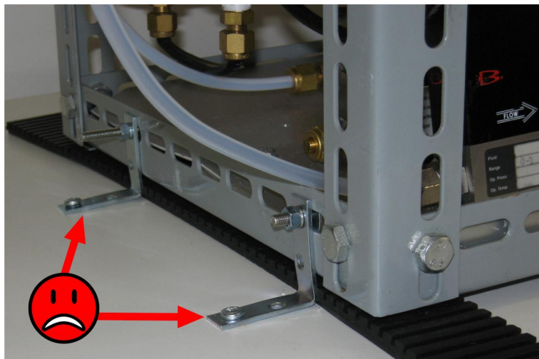
BILD 10. Plåtvinklar håller en vibrerande maskin på plats – men vinklarna leder även stömljud och detta är inte en bra lösning om det finns ljudkrav i rummet under eller vid sidan av. Maskinen borde ha skruvats fast i ett tungt fundament som dämpar rörelserna i maskinen. Mindre fundament ställs på vibrationsisolatorer som är avpassade till varvtal och egenvikt. (Bild från Vibratec AB).
