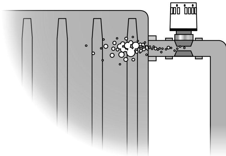
Bild 1. I trycksatta rörledningar skapas vibrationer av höga vattenhastigheter och stora tryckfall, exempelvis över radiatorventiler och liknande. Vibrationerna kan fortplanta sig till radiatorerna som i sin tur fungerar som "högtalare" när de vibrerar (luftljud).
