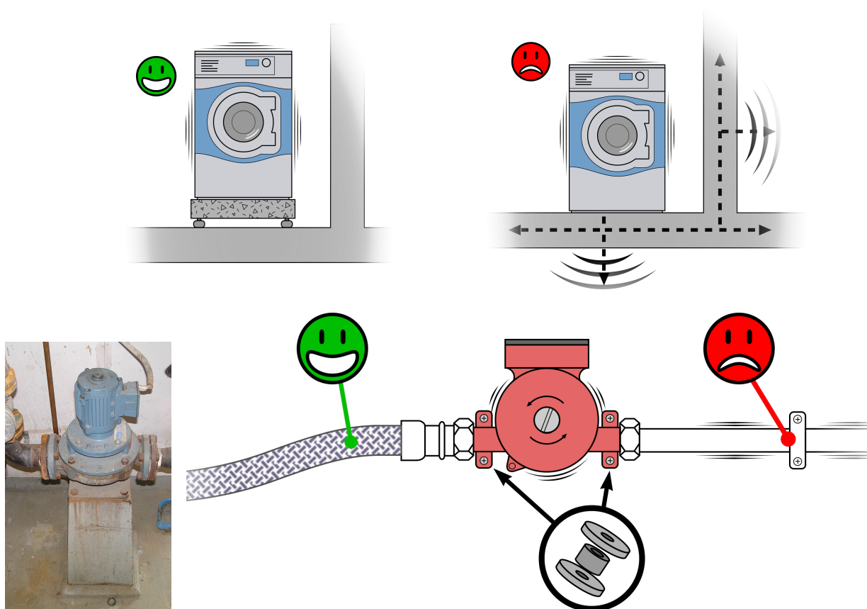
Bilder 4: a) Tvättmaskin med en tung bottenplatta och avpassade vibrationsisolatorer ger minimalt stomljud ned i ett betongbjälklag. b) Samma maskin som står på bjälklaget kan överföra stomljud. c) Större pumpar bör normalt monteras styvt i ett betongfundament, som placeras vibrationsisolerat mot bjälklaget. d) Mindre pumpar kan sättas fast med vibrationsisolerande plugg och anslutas elastiskt med gummikompensatorer eller stålspunna gummislangar. För alla maskiner med roterande delar som ställs på lätta bjälklag eller hängs upp i lätta väggar gäller att eventuella tilläggsåtgärder måste beskrivas av en sakkunnig (akustiker).
