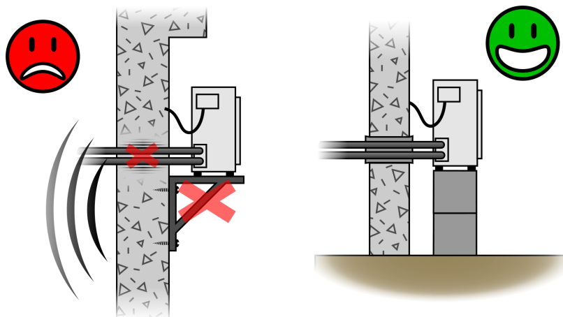
Bilder 13: Frånluftsvärmepumpar bör inte ställas bredvid eller över boningsrum där man har lätta bjälklag eller lätta väggar. Ljudproblem kan även uppstå vid placering utomhus, om kylmedelsrören är felklamrade, eller lindade med skumplastisolering som är för hård (PUR-skum) eller är för mjuk. Cellgummin (så kallad "kyltejp") trycks samman och blir hård redan efter en kort tid. Genomföringen ska isoleras med ett material som behåller sin elasticitet över tiden, exempelvis plastklädd mineralull eller ljudtejp. Kondensvatten ska avledas så att isbildning inte kortsluter rörelser i vibrationsisolatorerna.
