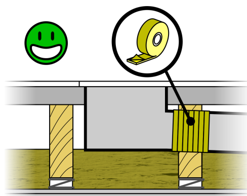
Bild 6. Vid montering av brunn och avloppsrör i bjälklag ovanför sovrum, vardagsrum, matrum och övriga rum med ljudkrav: a) Brunnen bör inte avvibreras utvändigt därför att rörelserna kan medföra läckage i tätskiktet. Välj istället en brunnprodukt som ger lågt stomljud (exempelvis i belagt gjutjärn med plastinsats) eller tilläggsisolera undersidan av bjälklaget. b) vid lätta bjälklag, montera brunnen styvt och vattentätt enligt leverantörens anvisningar. Svep de delar av brunn och avloppsrör som riskerar att ligga an stumt mot regler eller undertak med ljudtejp. Avpassa undertaket efter vilken brunn som används, inklädnader med mera.
