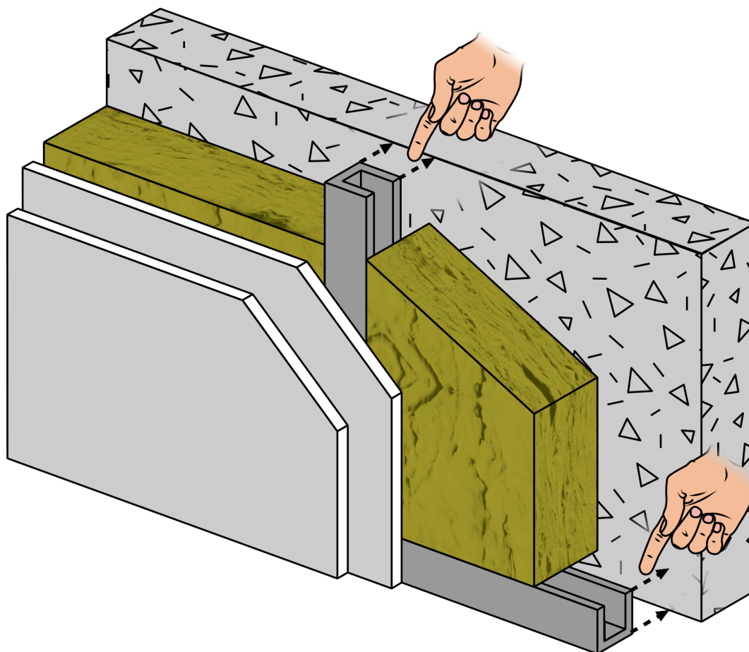
Bild 15. Tilläggsisolering med trä- eller stålreglar som står fritt cirka 25 mm ut från betongväggen, samt 70-95 mm mineralull och 2 lag skivor av gips eller motsvarande tungt skivmaterial. Fuktsäkra skivor ska användas om våtrumskraven anger detta. Kontrollera att reglarna står helt fritt från betongväggen innan skivorna sätts på plats.
