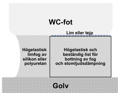
Bilder 12. Montering av WC på golv: a) utan dämpning, skruvad stumt i bjälklaget, b) med stomljudsdämpande list och fog, c) list och fog, d) fogad WC-stol på stomljudslist på plats [Formination: Bild c kommer som originalfil liknande tidigare figurer]
