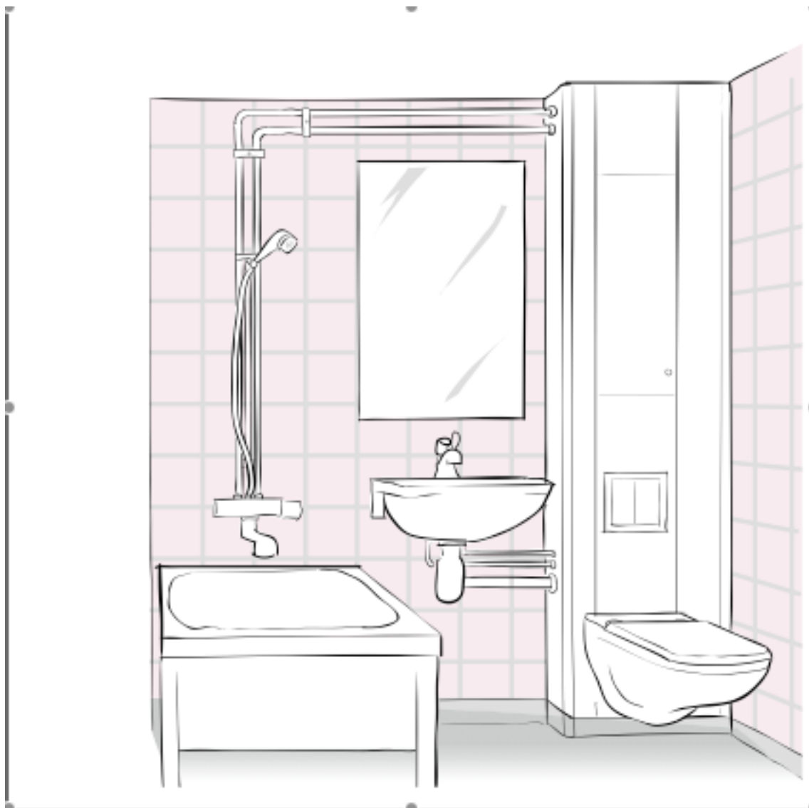
Bild 14. Tilläggsisolera väggar mot sovrum mm, där det inte är möjligt att avvibrera installationerna i våtrummet på den motsatta sidan. Formation, använd bilder från våtrumsskriften/ROT
