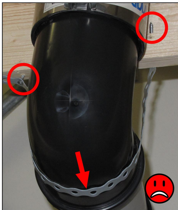
Bild 5: a) Skruva inte fast avloppsröret styvt i en bärande golvregel, b) Undvik styva kontaktpunkter mot stommen, särskilt nära riktningsändringar eller förgreningar. Vibrationerna i röret leds ned via skruvarna till bjälklaget och ger stomljud i detta.
